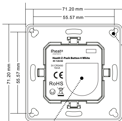
Parte posterioară
